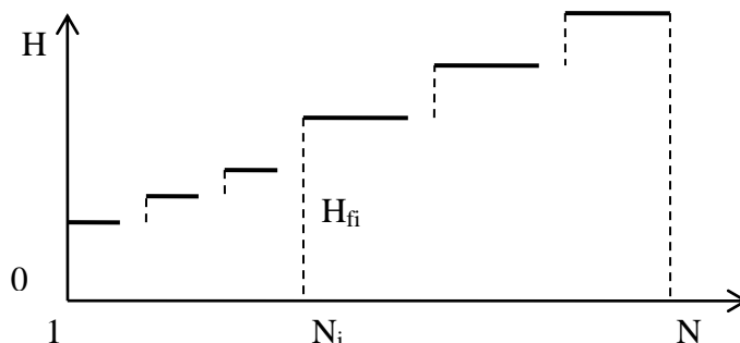
Рисунок 4 – Схема ступенчато-возрастающего режима приложения ударной нагрузки
