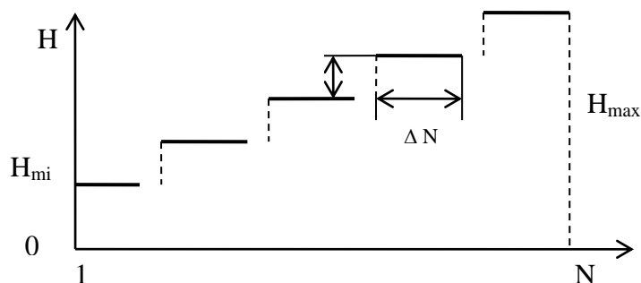
Рисунок 9 – Схема ступенчато-возрастающего режима приложения ударной нагрузки по грунту котлована
