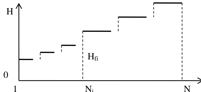
4 – сурет Соққы жүктемесінің баспалдақты- өсіре қолданылу тәртібінің сұлбасы
